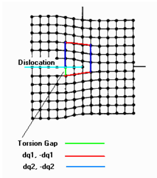
Edge dislocation gap due to Affine Torsion
